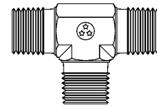
TMM - page 10 Té mâle Male Tee T-Einschraubverschraubung
